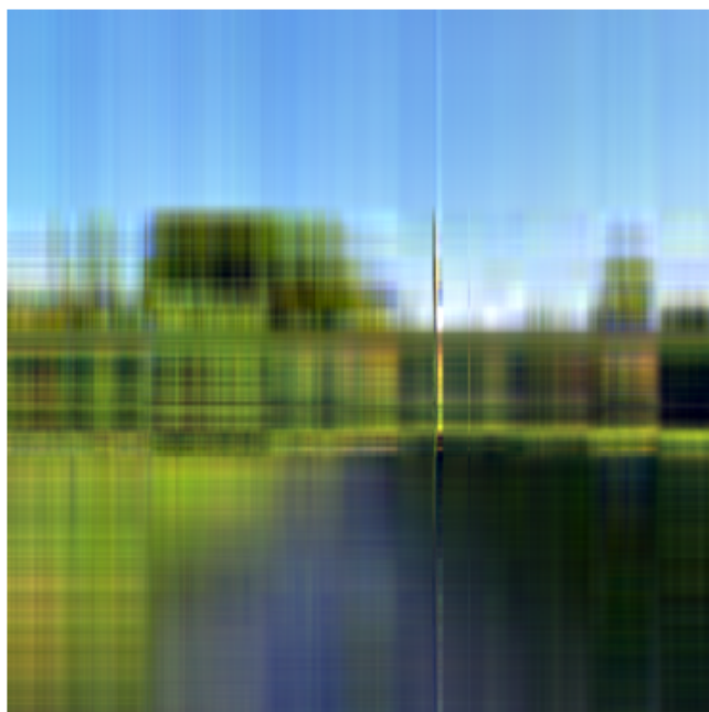
Slika 6.2: Rang r=5
