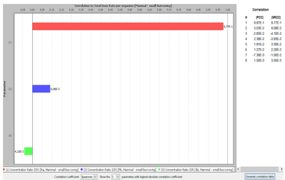
Slika 42. Dijagram tornada za male sisavce kopace
