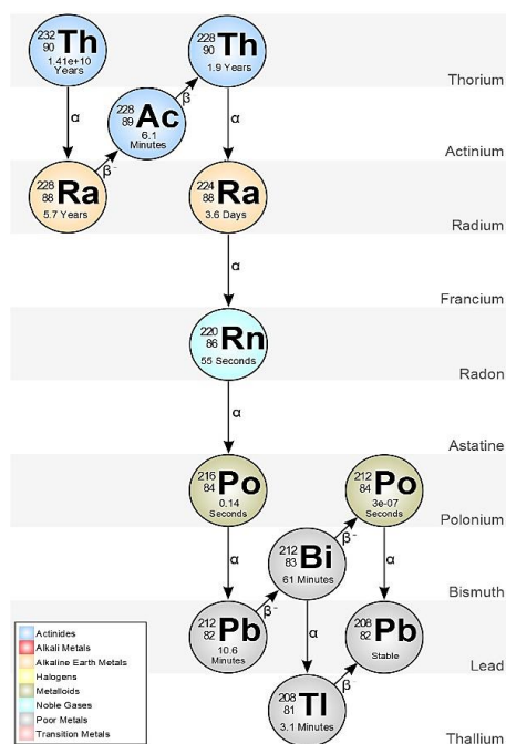
Slika 5. Lanac radioaktivnog raspada ^{232}\text{Th} 4
