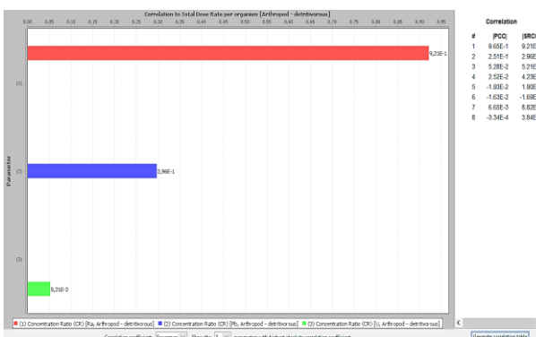
Slika 38. Dijagram tornada za člankonošce - detritivori
