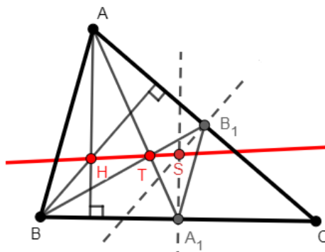
Slika 4. Eulerov pravac.
